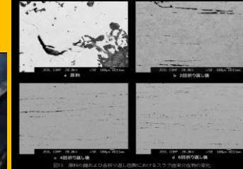
折り返し鍛造介在物 分布変化
