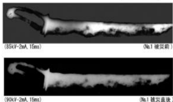
図1 調査した蕨手刀の外観とX線透過写真
