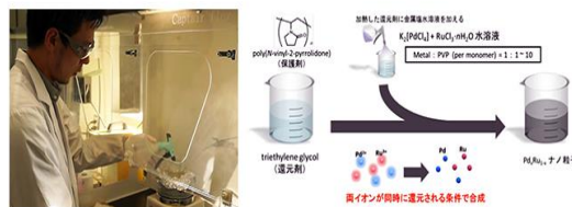
図3 液相還元法によるPdRu合金ナノ粒子の合成.
