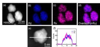
図5 Pd 0.5 Ru 0.5 合金ナノ粒子の状態観察. (a) HAADF-STEM像, (b) Pd-L線のマッピング, (c) Ru-L線のマッピング, (d) Pd-LとRu-Lの重ね合わせ, (e) 元素分析, (f) Pd-LとRu-Lの強度プロファイル.
