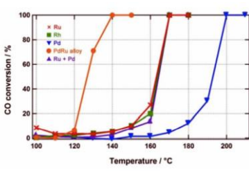
図5 γ-Al 2 O 3 に担持したナノ粒子のCO転換率の温度依存性 [13]。 ● Pd 0.5 Ru 0.5 合金、× 純Ru、■ 純Pd、▲ 純Pt、△ 純Pdと純Ptの物理混合。
